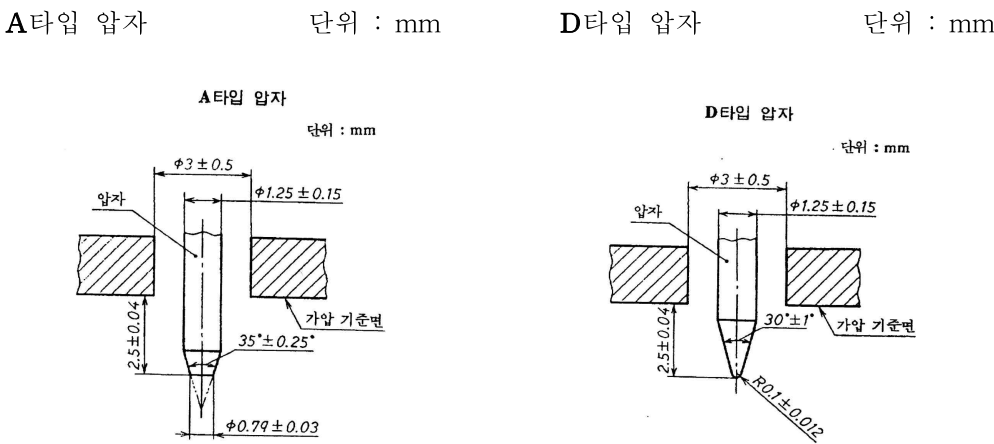
<그림 1> 듀로미터 압자의 모양 및 치수
